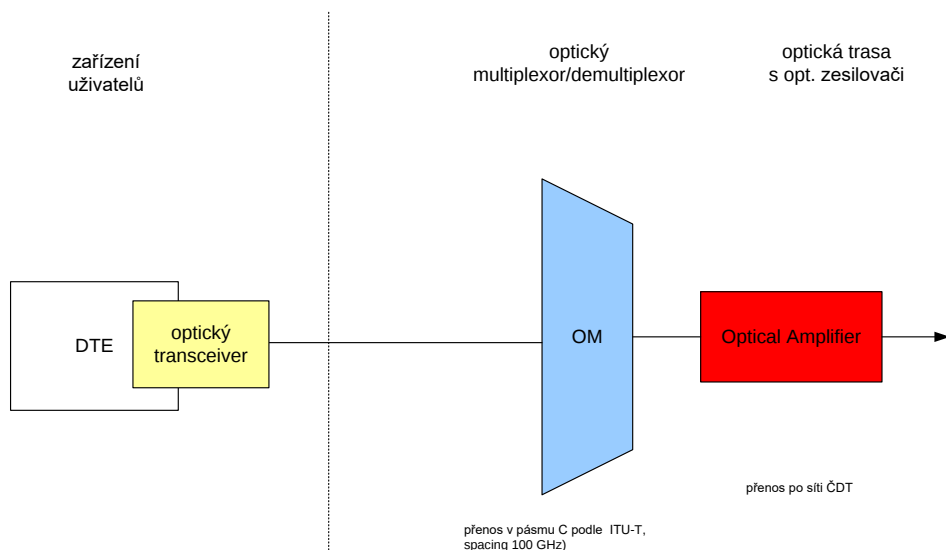
Obrázek č.2 – využití optických transceiverů
